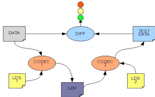
Figure 11. Schéma de mise à l'épreuve.
