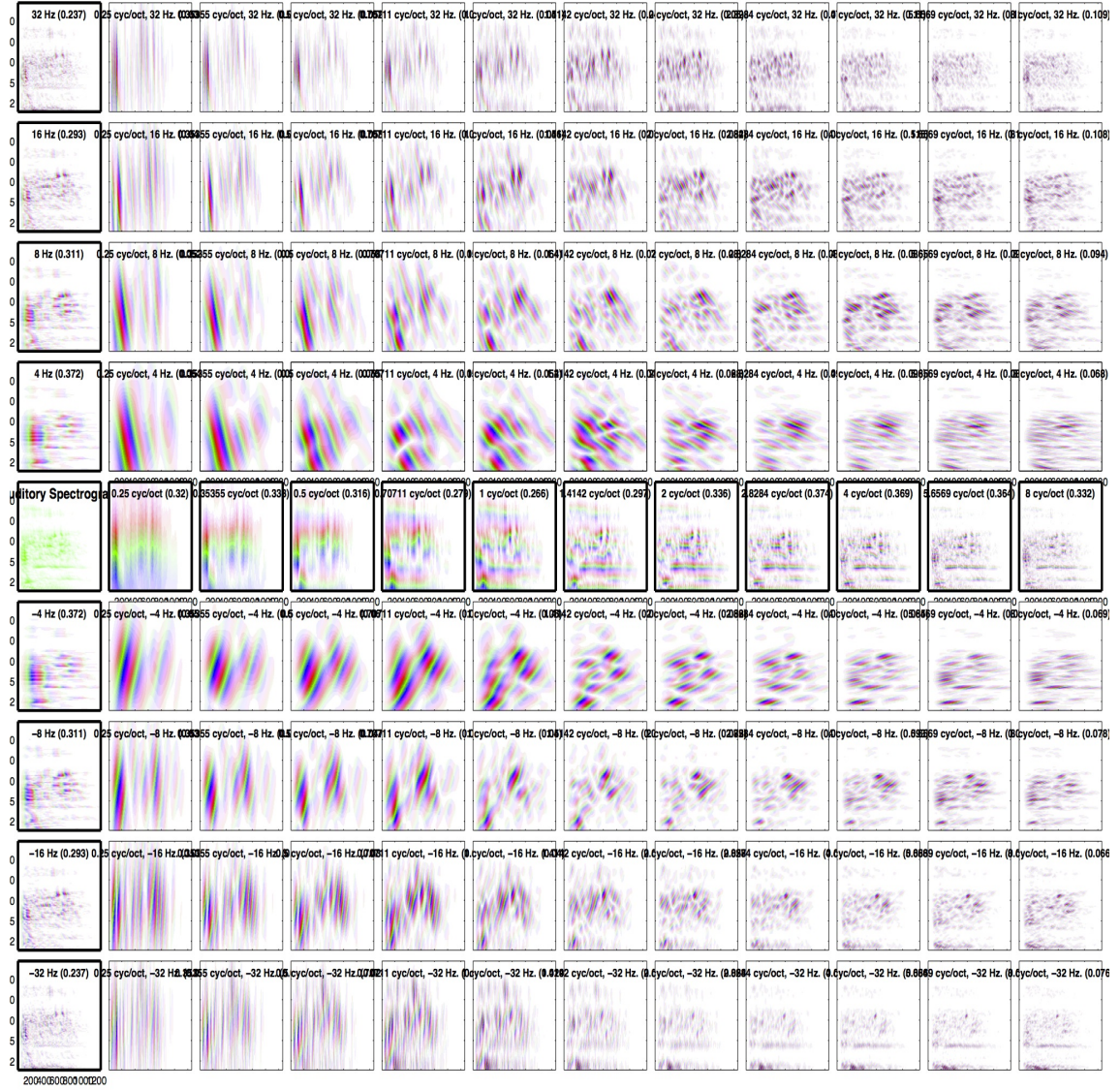
FIGURE 2.1 – Représentation corticale d'un son de rugissement de lion.
